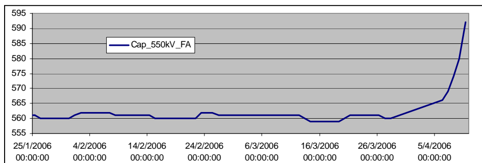
Figura 8 – Aumento de la Capacitancia en el bushing de 550kV del autotransformador de la fase A
