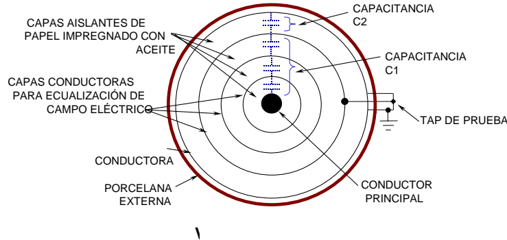
Figura 1 – Forma constructiva de un bushing condensivo
