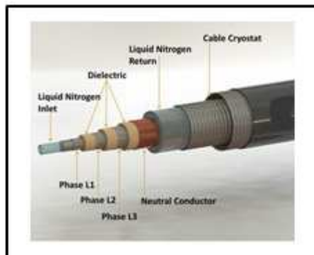
Figura 6. El cable concéntrico superconductor se enfría con \text{N}_2 líquido (Foto: Nexans) [12].
