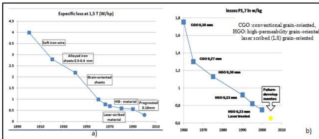
Figura 3: Evolución del material del núcleo de transformador [2].
