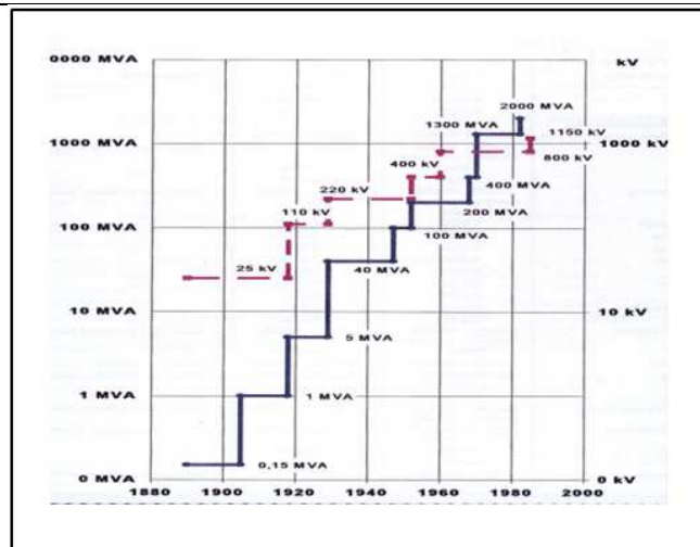
Figura 1: Evolución del voltaje y la potencia de transformadores [2].
