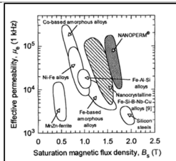
Figura 8. Comparación de materiales magnéticos blandos tradicionales (indicados sin relleno) con los nuevos materiales magnéticos amorfos y nano cristalinos (regiones con distintos rellenos) [14].
