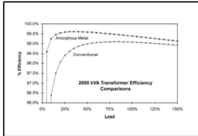
Figura 7. Eficiencia entre un transformador de núcleo convencional y uno de núcleo amorfo [14].
