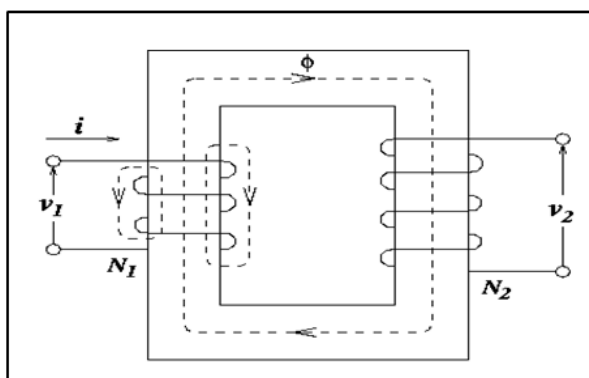
Figura 2: Diagrama esquemático do transformador
