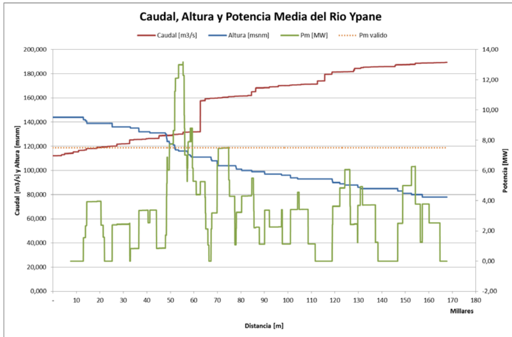
Figura 7. Potencial Hidroenergético con L = 7,5 km
