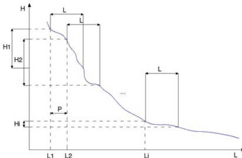
Figura 4. Esquema del proceso de búsqueda del potencial Hidroenergético utilizando una ventana móvil
