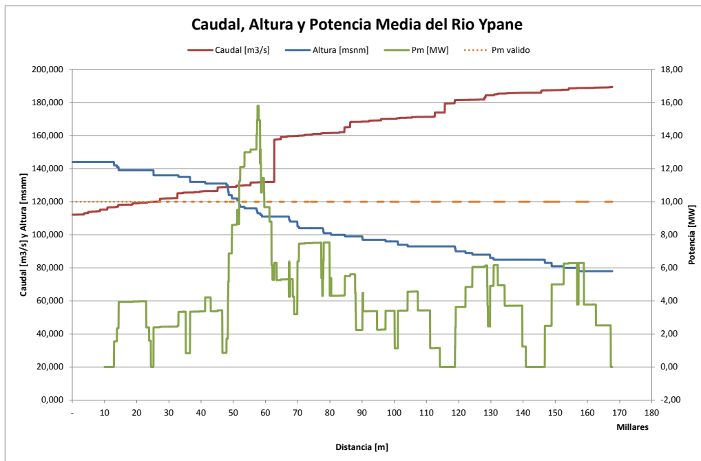
Figura 8. Potencial Hidroenergético con L = 10 km
