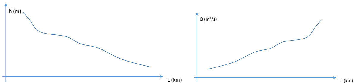
Figura 3. Curvas de Perfil Longitudinal del Río y Potencial Hidráulico
