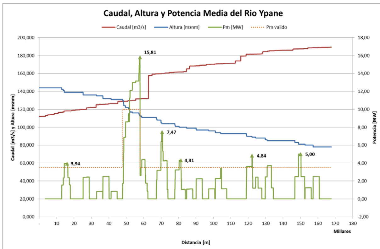
Figura 9. Potencial Hidroenergético identificado en el Río Ypané
