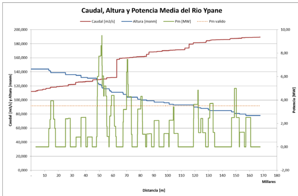
Figura 5. Potencial Hidroenergético con L = 3,5 km
