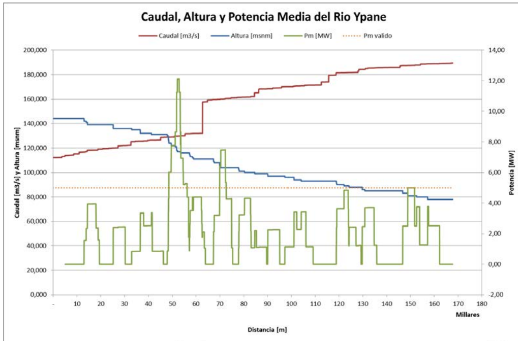
Figura 6. Potencial Hidroenergético con L = 5 km
